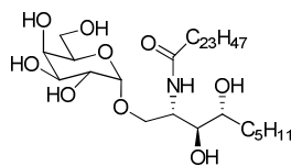
Figure 3: Structure of OCH
